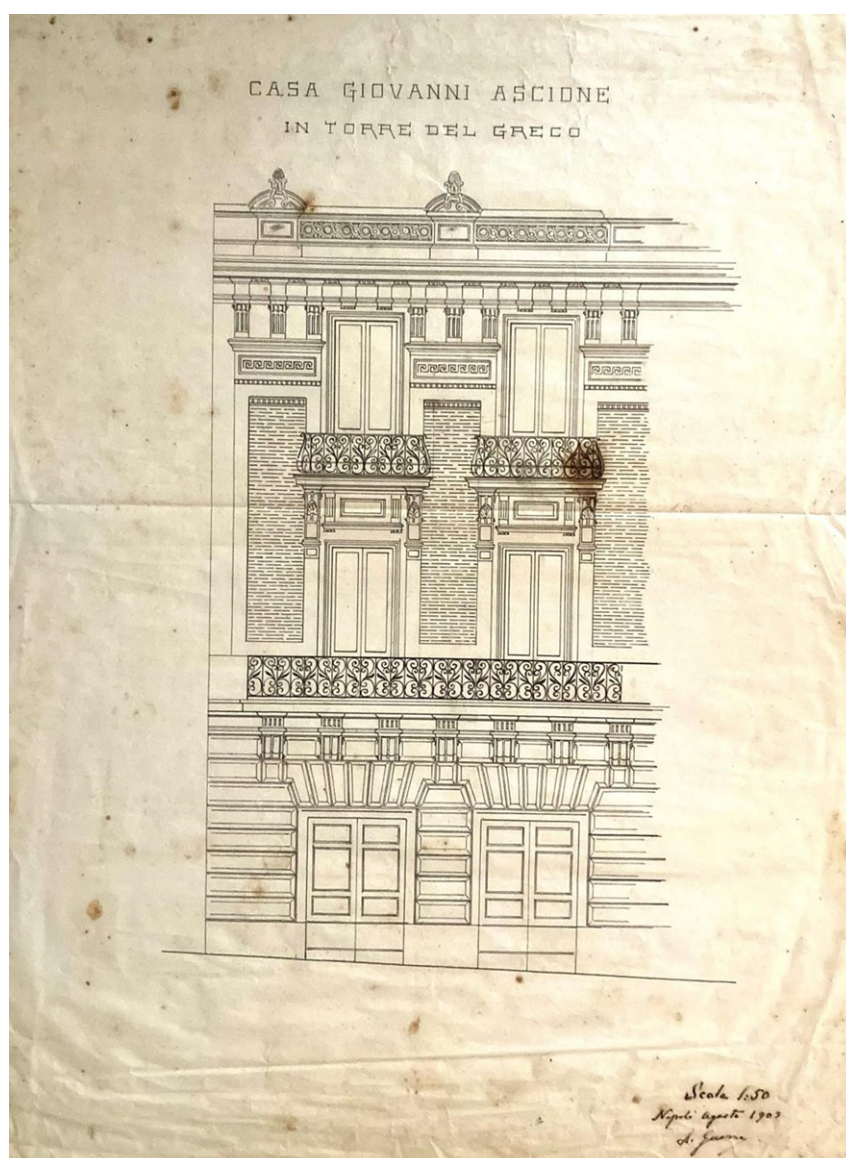
Progetto di Alfonso Guerra del palazzo Ascione di Torre del Greco, Napoli, agosto 1905 (Sede di Torre del Greco, Fondo iconografico, Casa Giovanni Ascione in Torre del Greco, cartella 1)
